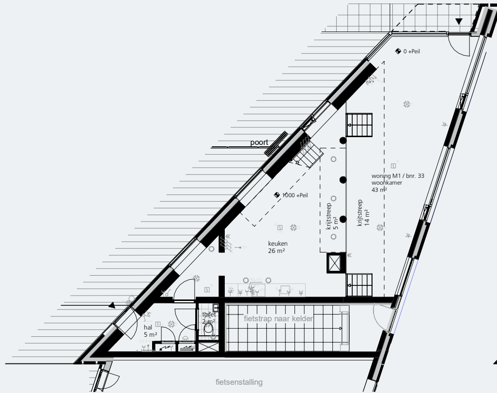
begane grond
