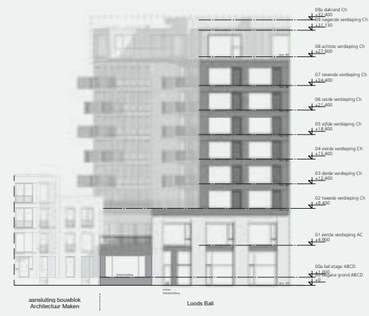
aansluiting bouwblok Architectuur Maken Loods Ball
